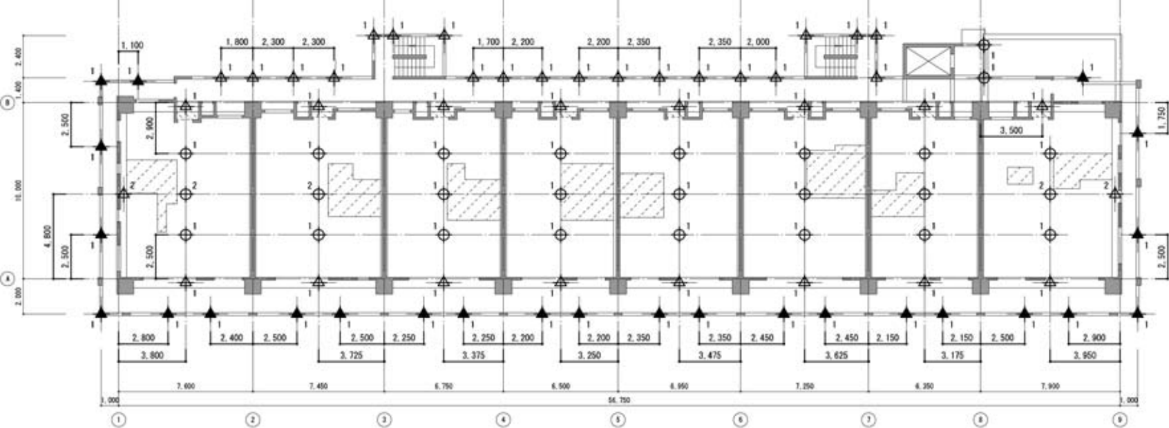
2階床梁クイックサポート配置図 (見下げ) 1:200
